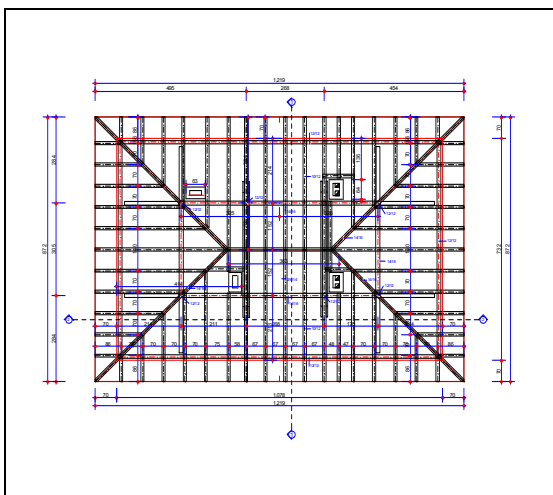
основа крова
