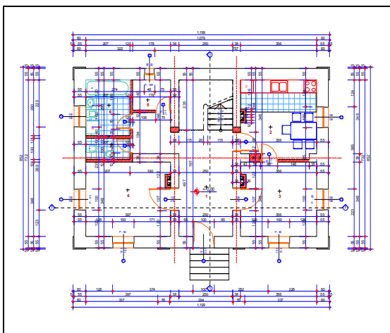
основа приземља
