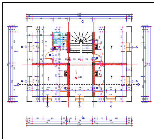
основа спрата
