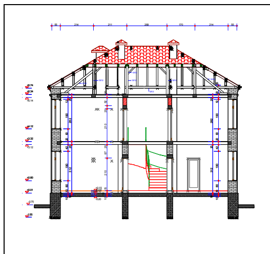
подужни пресек
