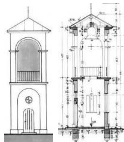
Детаљи пресека звоника
